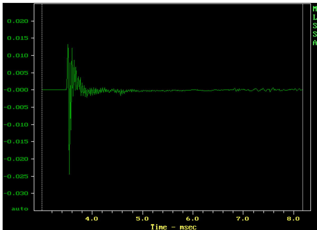
6. Переходная характеристика
